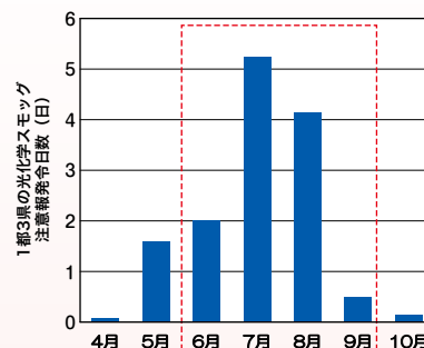
光化学スモッグ注意報 月別発令状況 (平成26年度～令和5年度平均値)
